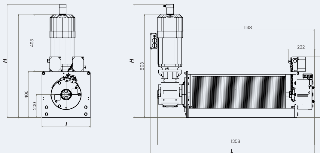
Dimensions du TRDI500 à 6 câbles, course 20 mètres, moteur vertical
